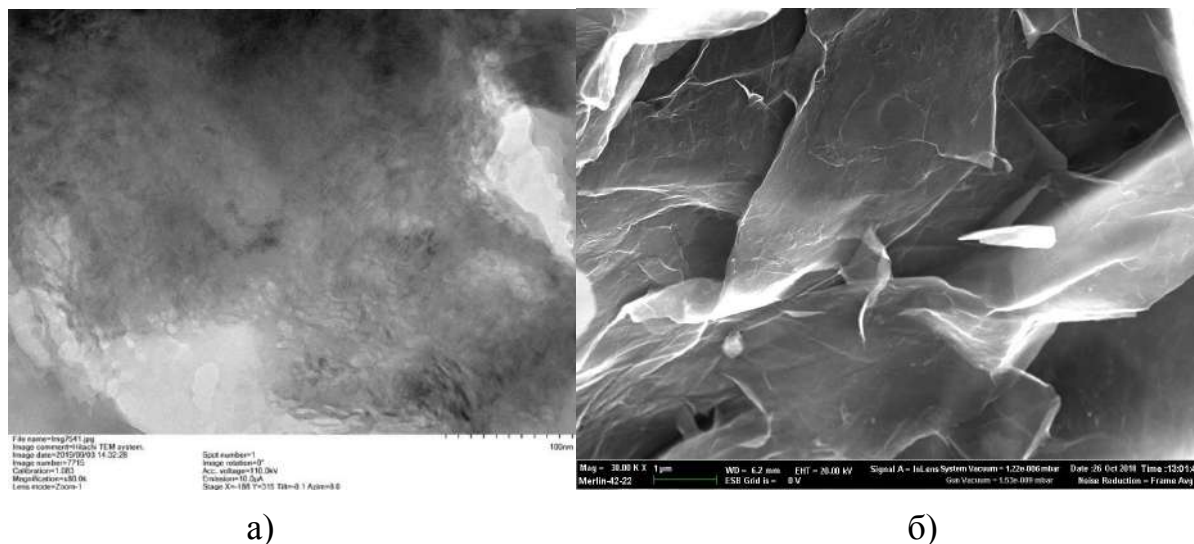
Рис. 1. Снимки частиц коллоидного графита, полученные методами просвечивающей (а) и сканирующей (б) электронной микроскопии.
