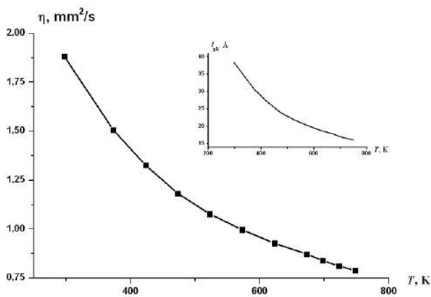
Рис. 2. Температурная зависимость температуропроводности \eta ТРГ. На вставке температурная зависимость средней длины свободного пробега фононов l_{ph} .
