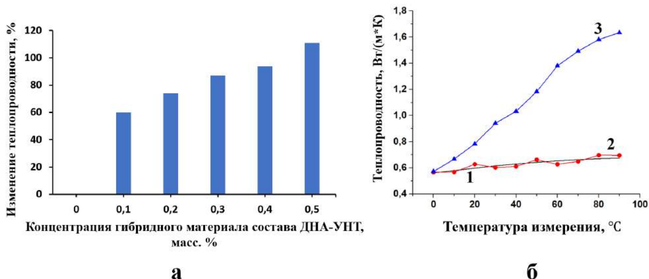
Рис. 3. Теплофизические свойства наножидкости на основе воды, модифицированной гибридным материалом ДНА-УНТ. а – зависимость теплопроводности наножидкости от концентрации гибридного материала (при 50 °С); б - зависимость теплопроводности наножидкости от температуры измерения где 1 – теплопроводность воды (справочные данные), 2 - теплопроводность воды (экспериментальные данные), 3 – теплопроводность наножидкости с 0,5 масс. % гибридного материала.
