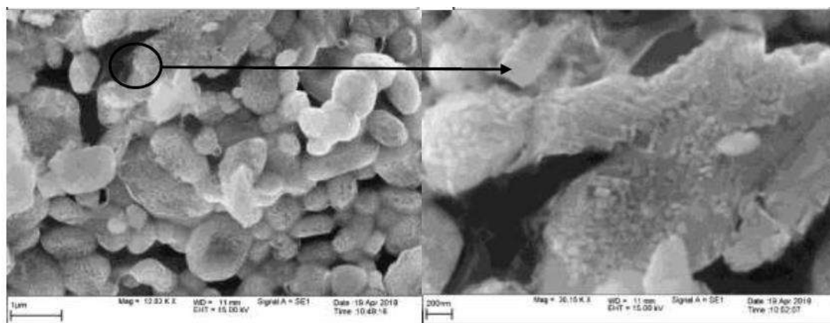
Рис. 1. Изображение СЭМ частиц диборида циркония.
