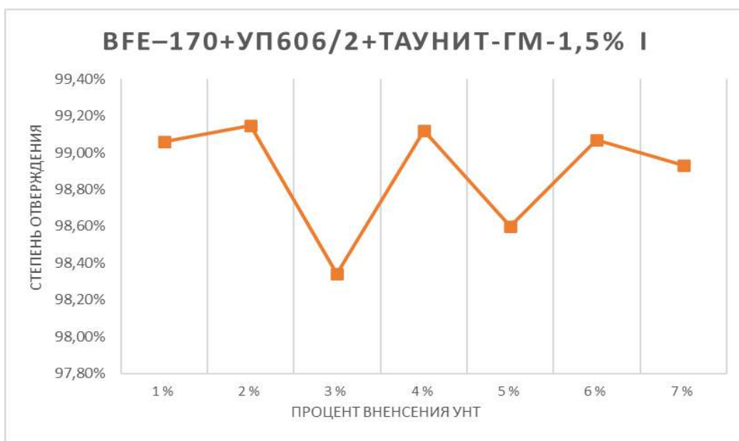
Рис. 1. Влияние концентрации УНТ «Таунит-ГМ», обработанных йодом (1,5 %) на степень отверждения эпоксидной смолы ВFE-170 с отвердителем УП606/2
