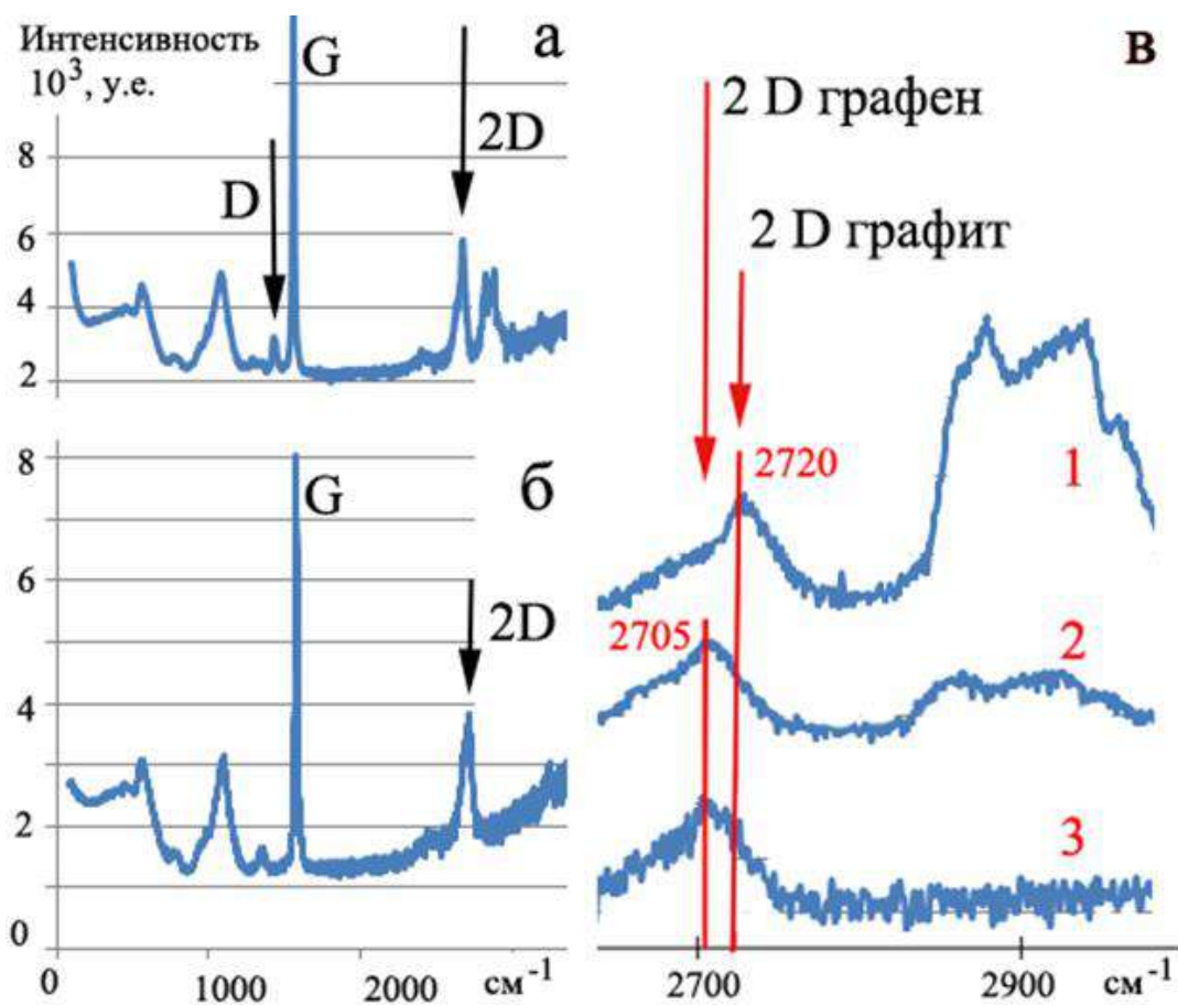
Рис. 3. PC суспензий, содержащих графен до «взрывной» эксфолиации (в1) и после (а, б, в3); растворители керосин (а, в1, в2), этиловый спирт (б, в3);
