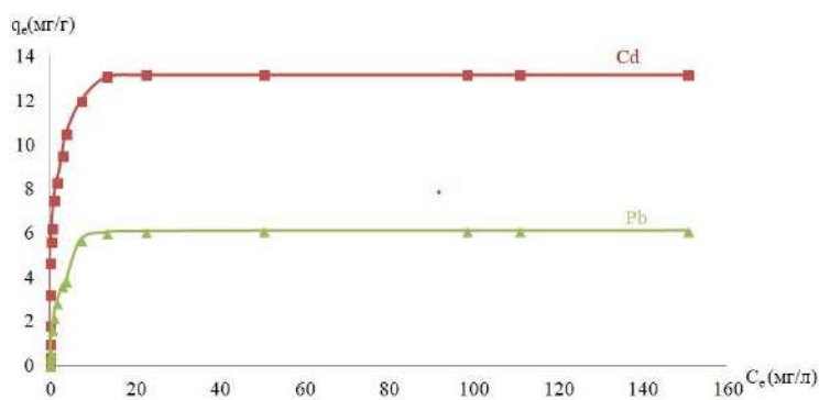
Рис. 2. Изотерма адсорбции Cd (II) и Pb (II) термовосстановленным оксидом графена.
