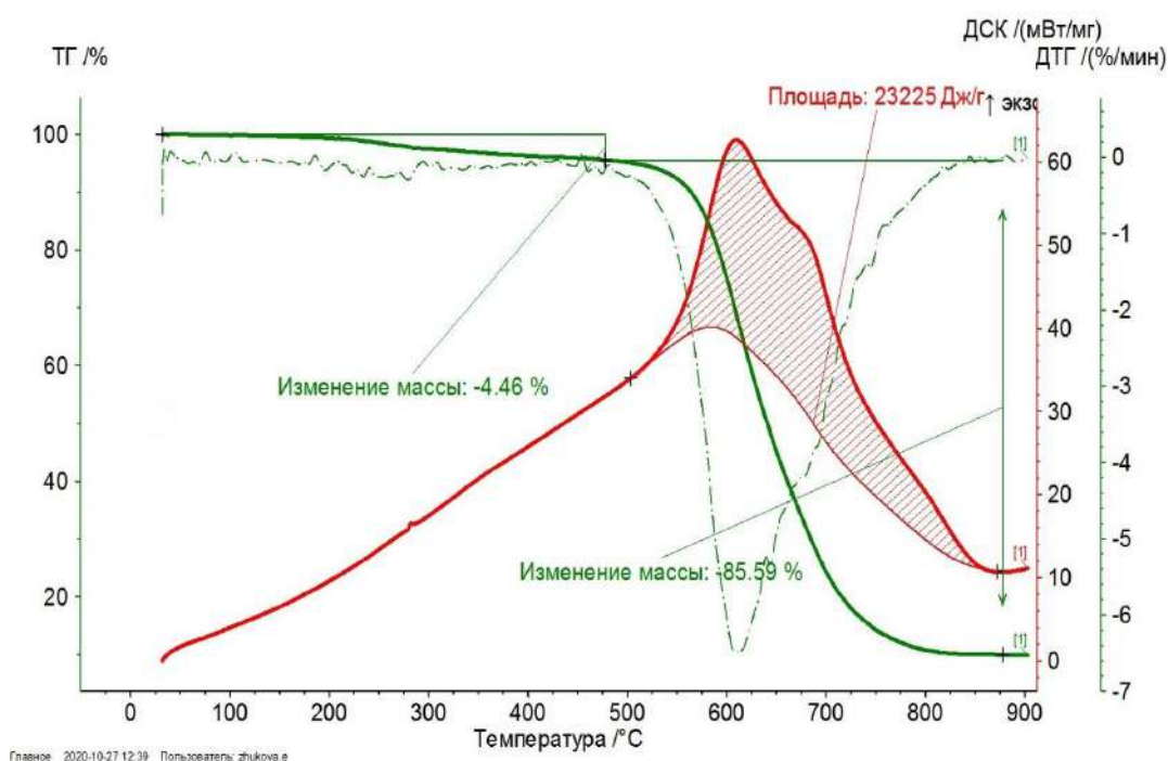
Рис. 1. Результаты ТА образцов УНТ, полученных из этанола в окислительной атмосфере (синтетический воздух – 50 мл/мин, гелий – 20 мл/мин): ТГ кривая (зеленый), ДТГ кривая (зеленый пунктир) и ДСК-кривая (красный).
