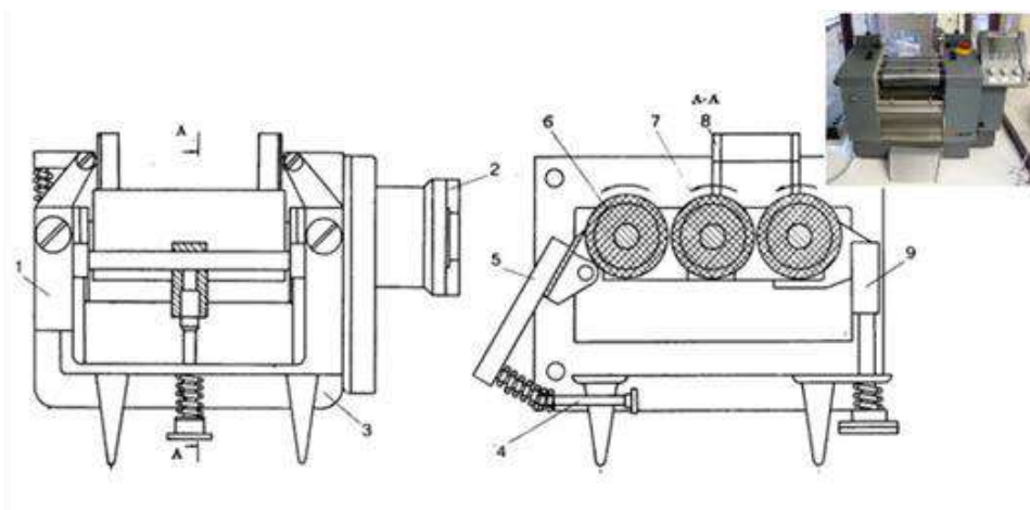
Рис. 1. Схема трехвалковой машины ЕХАКТ [8]. 1 – корпус подшипников; 2 – полумуфта; 3 – станина; 4 – поджим; 5 – скребок; 6, 7 – валок; 8 – бункер; 9 – регулятор зазора.
