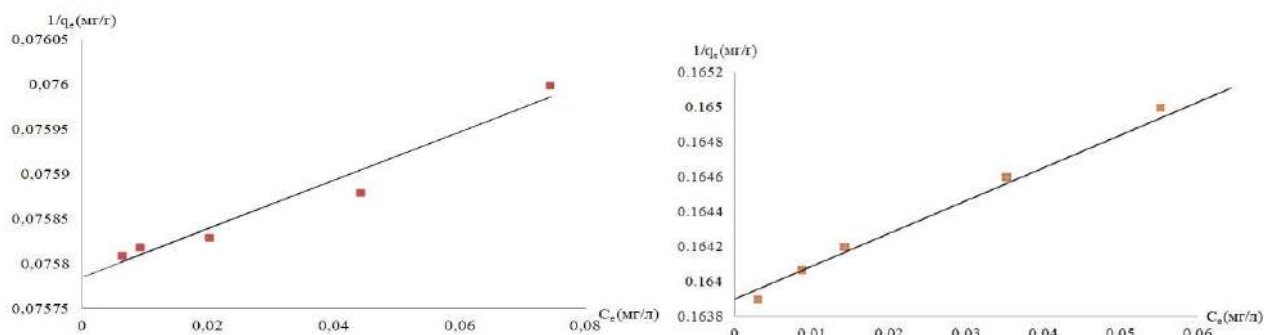
Рис. 3. Изотермы адсорбции Cd (II) (а) и Pb (II) (б) термовосстановленным оксидом многослойного графена, Ленгмюра.
