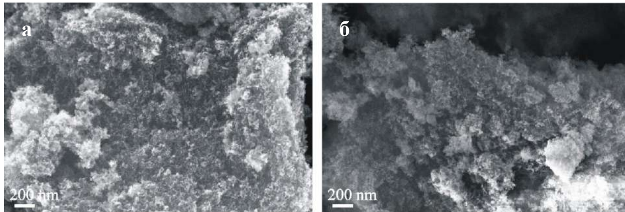
Рис. 1. СЭМ-изображения нанопорошков алмазной шихты, обогащенной бором, полученной подрывом заряда тротила с гексогеном (а) и тетрила (б).
