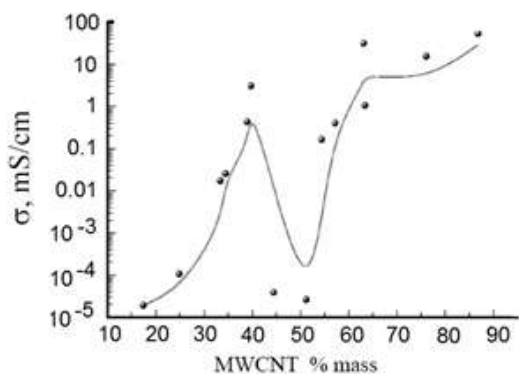
Рис. 3. Концентрационная зависимость электропроводности композита на основе МСУНТ и полимера.
