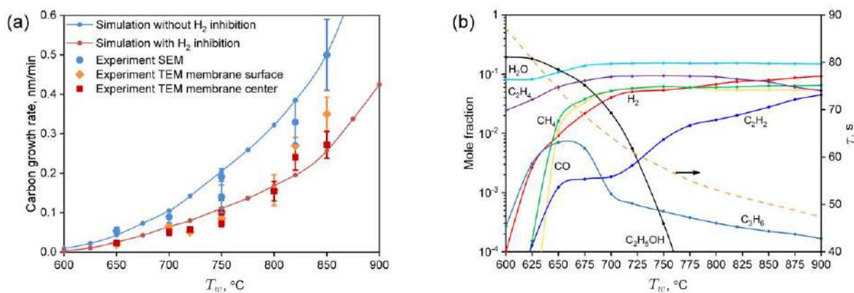
Рис. 2. Зависимость скорости роста стенок углеродных нанотрубок (а) и мольных долей частиц, усредненных по поверхности мембраны/времени пребывания (b) от температуры стенки реактора. Давление 0.5 бар, расход аргона 200 мл/мин, расход этанола 0.083 мл/мин.
