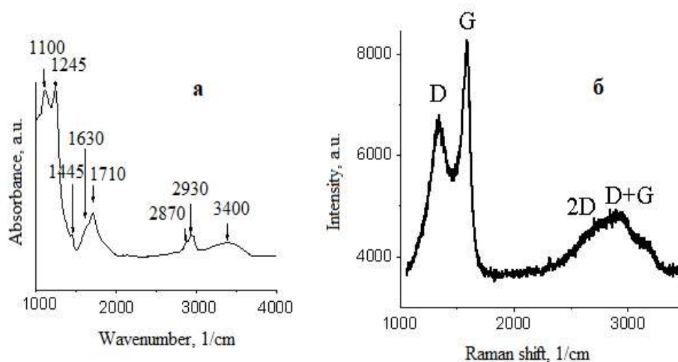
Рис. 1. Спектры поглощения в ИК-области (а) и Раман спектры (б) углеродных пленок, осажденных в плазме метана мощностью 200 Вт длительно-стью 9 мин и отжига при 650\text{ }^{\circ}\text{C} в течение 30 мин.
