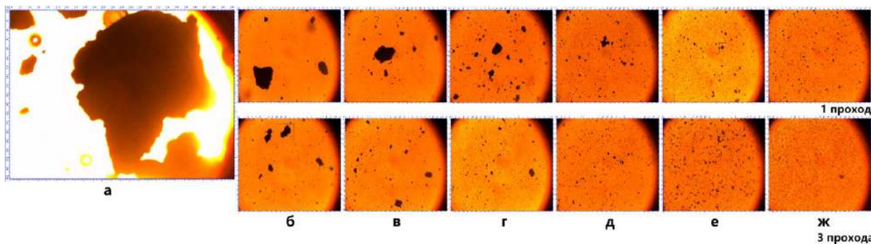
Рис. 2. Микроизображения образцов полимерной системы «УНТ-ЭД20», полученных при различных режимах обработки трехвалковой машины «ЕХАКТ». а – ручная обработка; б – мех. обработка при размерах зазора 60/30 мкм; в – при размерах зазора 30/15 мкм; г – при размерах зазора 15/15 мкм; д) – при усилии 4:4 Н/мм; е – при усилии 6:6 Н/мм; ж – при усилии 8:8 Н/мм.
