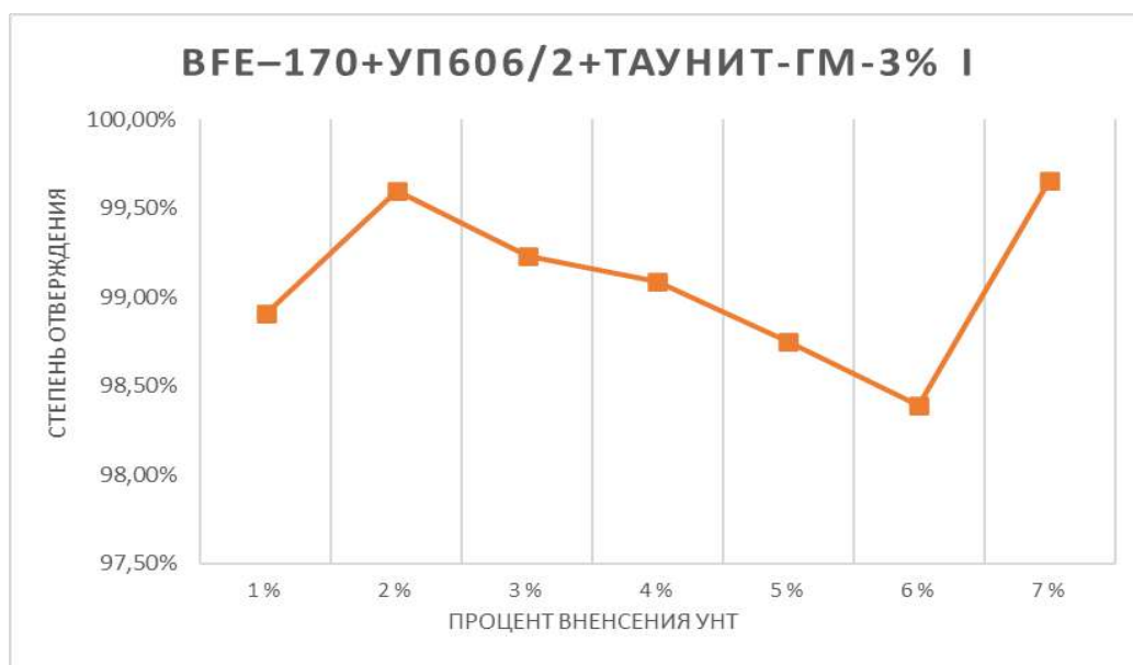
Рис. 2. Влияние концентрации УНТ «Таунит-ГМ», обработанных йодом (3 %) на степень отверждения эпоксидной смолы ВFE-170 с отвердителем УП606/2.
