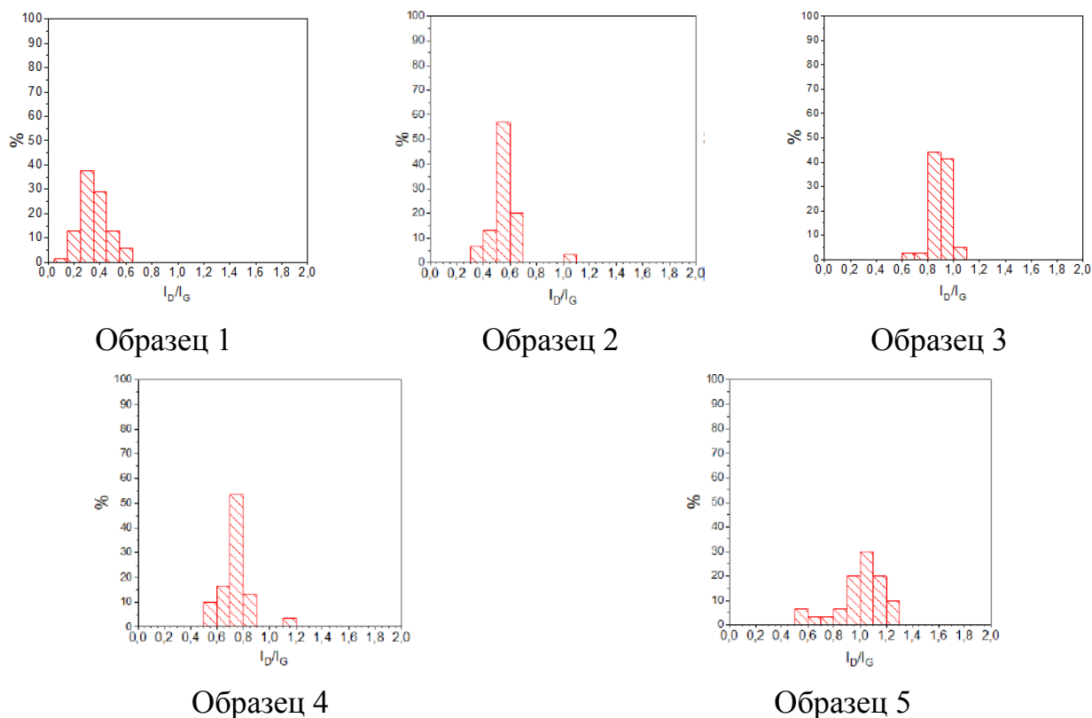
Рис. 2. Гистограмма распределения параметра I_D/I_G для исследуемых образцов.
